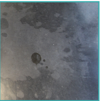
Um derramamento de refrigerante deixado em repouso por quase uma hora iluminou significativamente o concreto deste piso de concreto.
